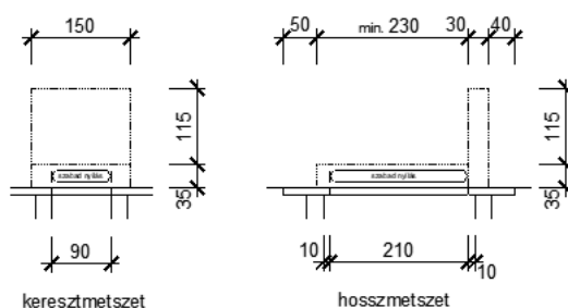
Különálló sírboltra építhető emlékmű maximális befoglaló méretei
