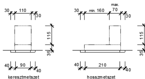
Felnőtt sírhelyre építhető emlékmű maximális befoglaló méretei, új parcella esetén
