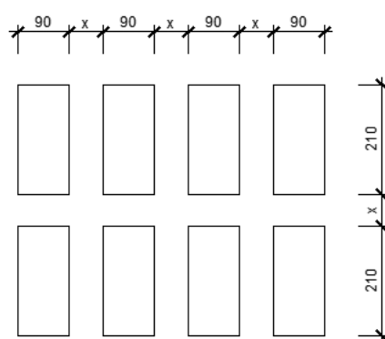
Felnőtt sírhely méretei, egymástól való távolsága
