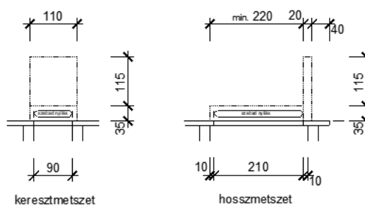
Különálló sírboltra építhető emlékmű maximális befoglaló méretei
