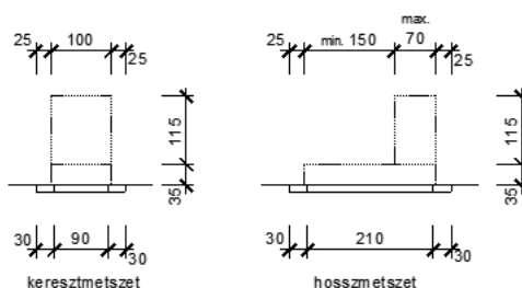
Felnőtt sírhelyre építhető emlékmű maximális befoglaló méretei meglévő, működő parcella esetén
