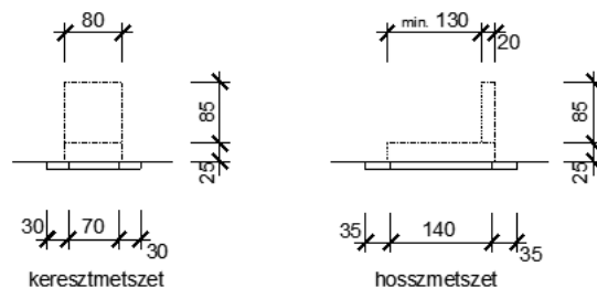
Gyermek sírhelyre építhető emlékmű maximális befoglaló méretei
