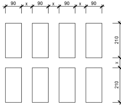
Felnőtt sírhelyre építhető járda méretei
